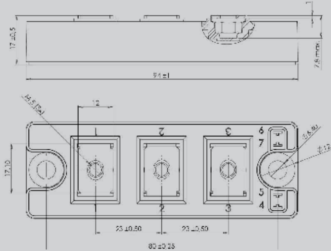
D1P
