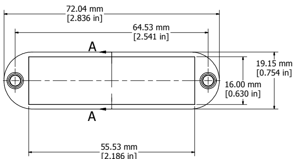
BEZEL
