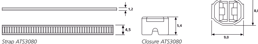
Strap ATS3080
