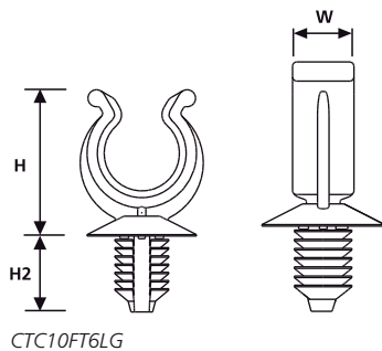
CTC10FT6LG
