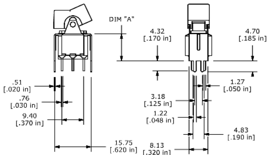
VS2-VS3 Termination - DP
