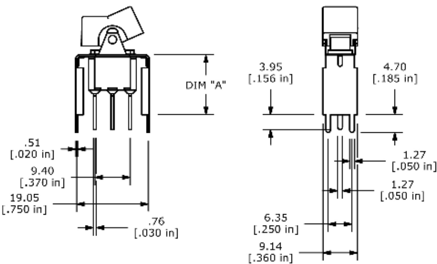
VS4-VS5 Termination - SP
