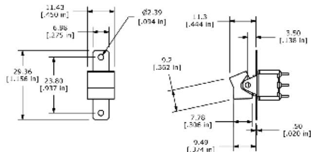
R11 Actuator
