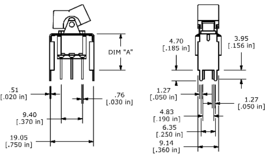
VS4-VS5 Termination - DP
