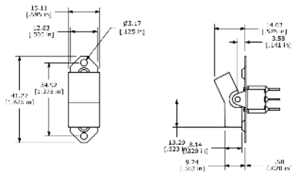
R3 Actuator
