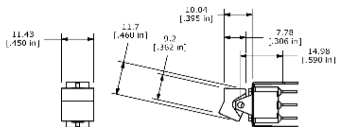
J5 Actuator
