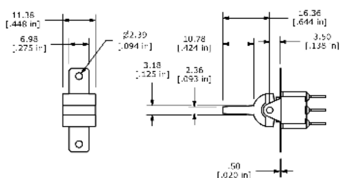
R16 Actuator
