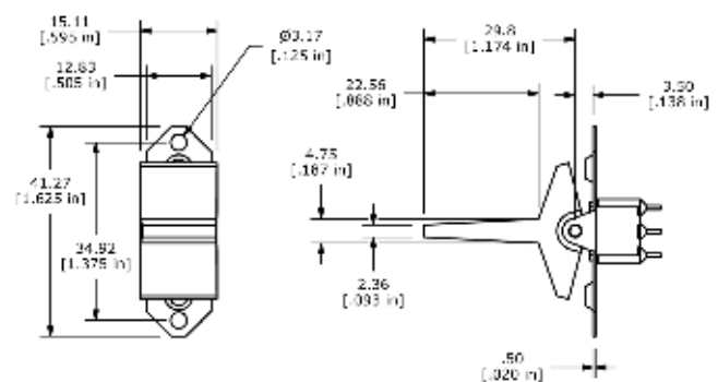
R4 Actuator
