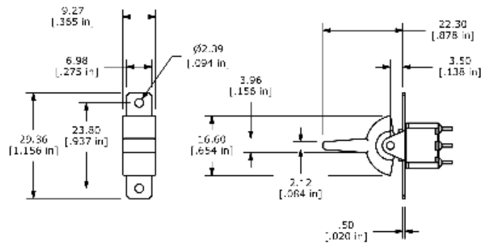
R2 Actuator
