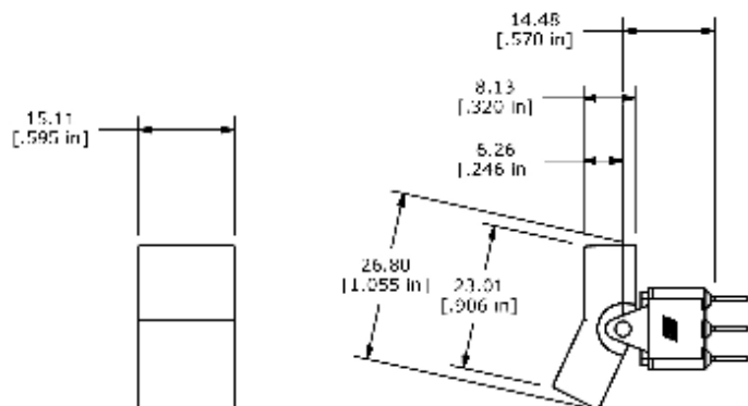
J3 Actuator
