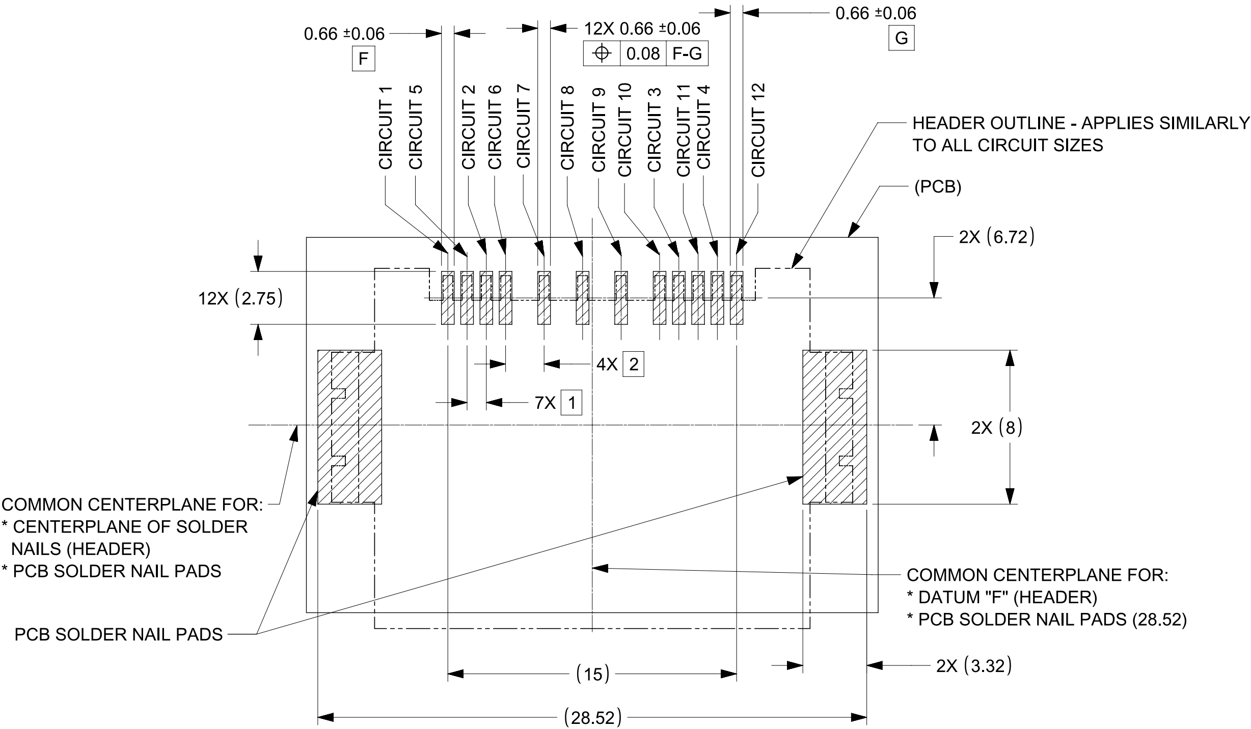
12 CKT PCB LAYOUT
