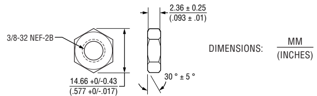
NUT H-38-2
