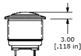
DOMED ACTUATOR
