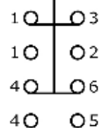
DPDT Non ILL. SCHEMATIC
