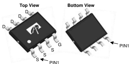
SOIC-8
