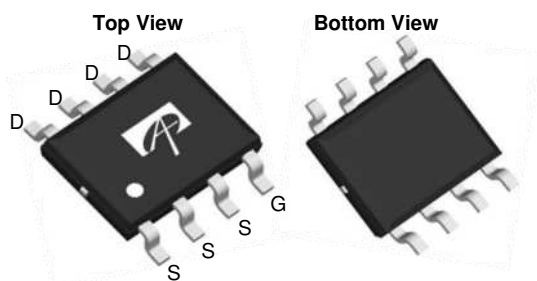
SOIC-8
