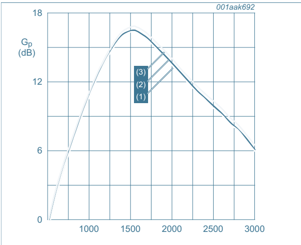
P_i = -45\text{ dBm} ; T_{amb} = 25\text{ }^{\circ}\text{C} . (1) V_{CC} = 1.5\text{ V} (2) V_{CC} = 1.8\text{ V} (3) V_{CC} = 2.85\text{ V}
