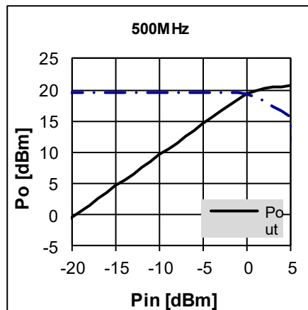
500MHz, 5V/85mA
