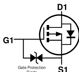
Q1 P-CHANNEL
