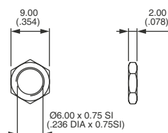
HEX NUT
