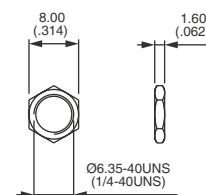
HEX NUT
