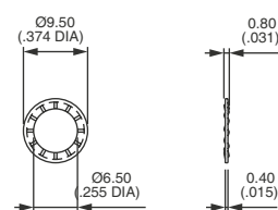
LOCKWASHER
