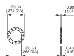
LOCKWASHER
