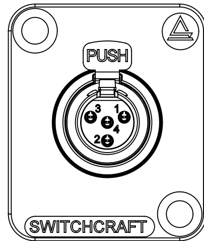
EHT4F 4 PIN
