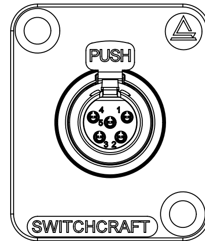
EHT5F 5 PIN
