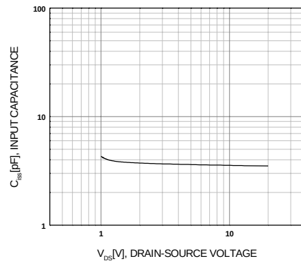
Figure 6. C_{iss} - V_{DS}
