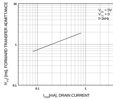
Figure 4. |y_{FS}| - I_{DSS}
