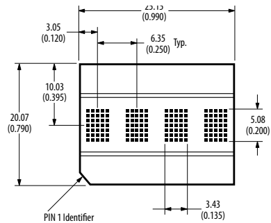
HDLx-2416
