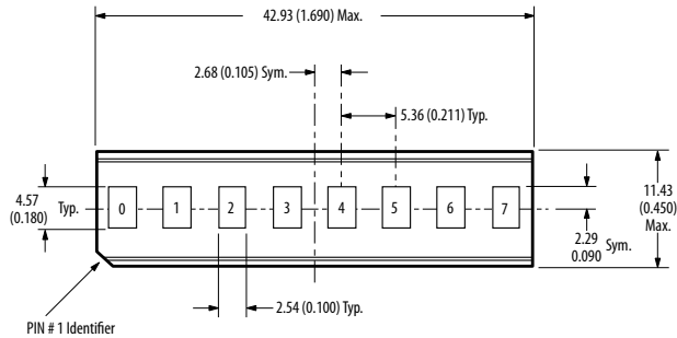
HDSP-253x
