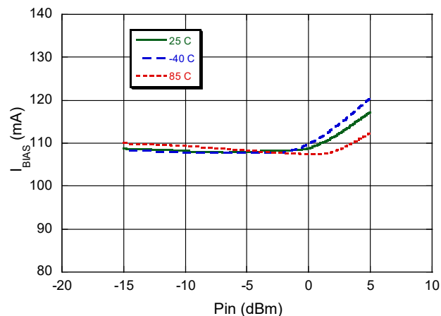
I_{BIAS} @ 15 GHz
