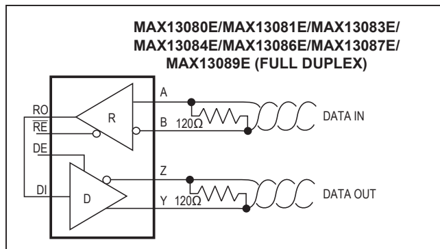
Figure 11. Line Repeater for MAX13080E/MAX13081E/ MAX13083E/MAX13084E/MAX13086E/MAX13087E/ MAX13089E in Full-Duplex Mode
