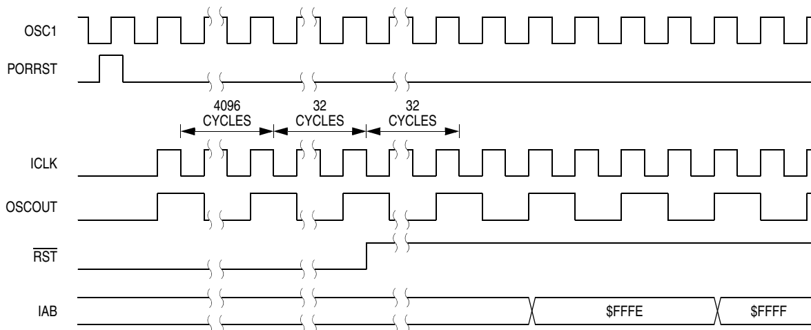
Figure 5-7. POR Recovery
