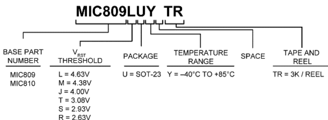
MIC809 SOT-23
