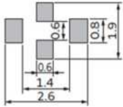
NFM21CC NFM21HC NFM21PC
