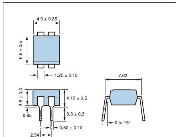
DIP4 Thru-Hole
