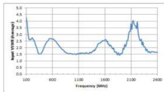
VSWR
