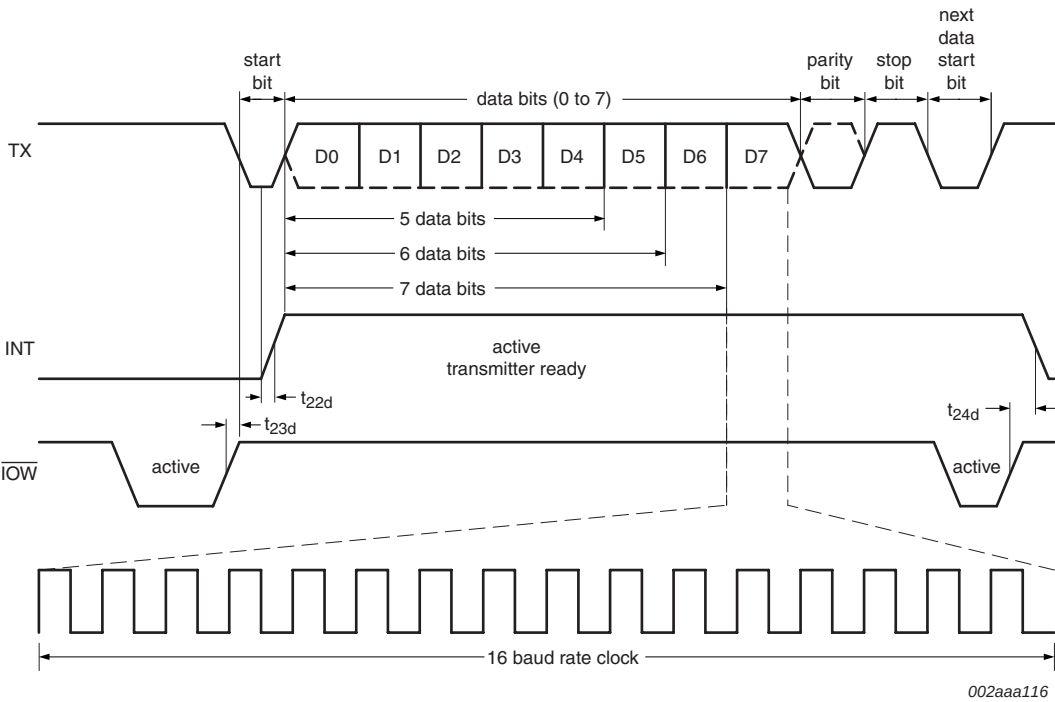
Fig 27. Transmit timing
