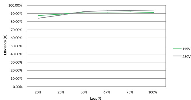
GCU500PS48
