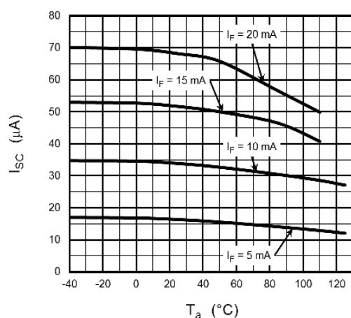
Fig. 12.9 I_{SC} - T_a
