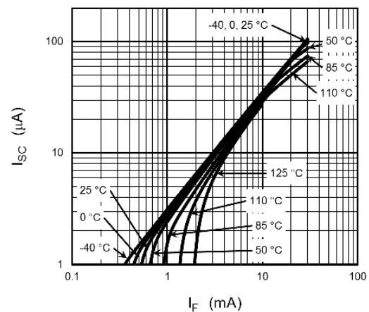
Fig. 12.6 I_{SC} - I_F
