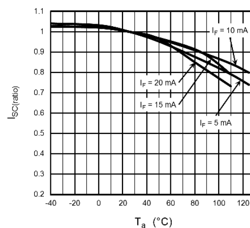
Fig. 12.10 I_{SC(ratio)} - T_a
