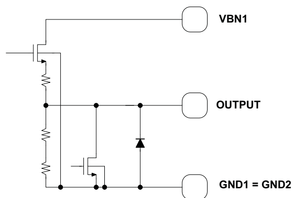
Figure 54. VREF1/VREF2
