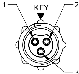
FACE VIEW W18280-3SG-P-3XX
