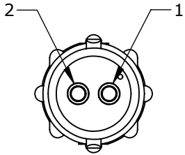
WIRING VIEW W18280-2SG-P-3XX
