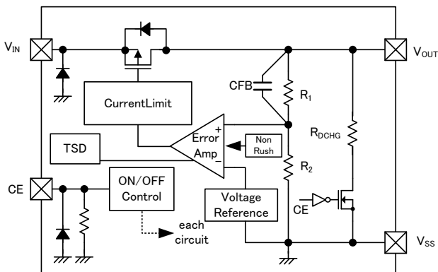
XC6223H/T
