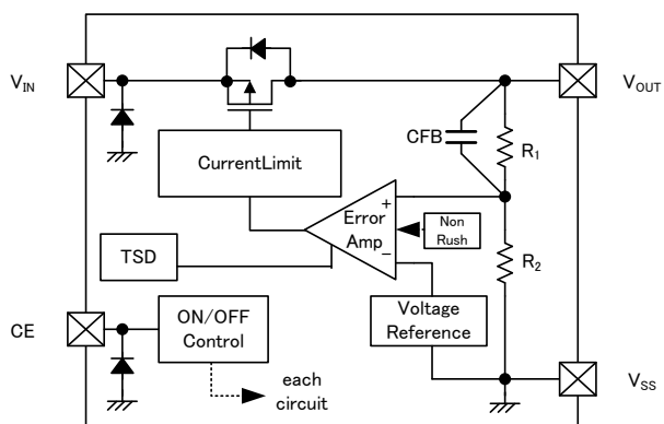
XC6223E/P
