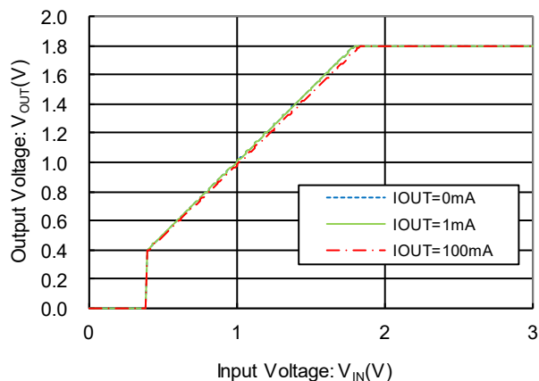
XC6602x181xR-G
