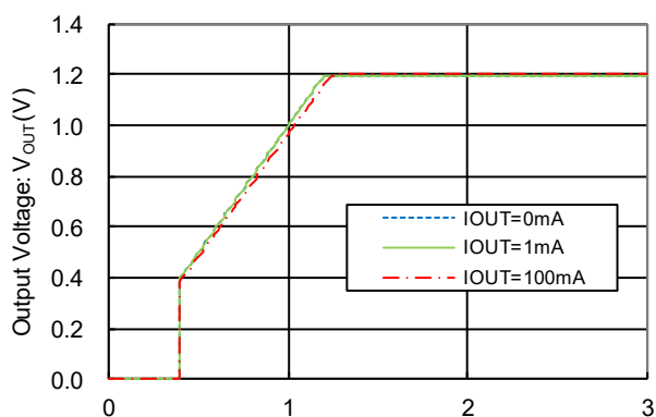
XC6602x121xR-G
