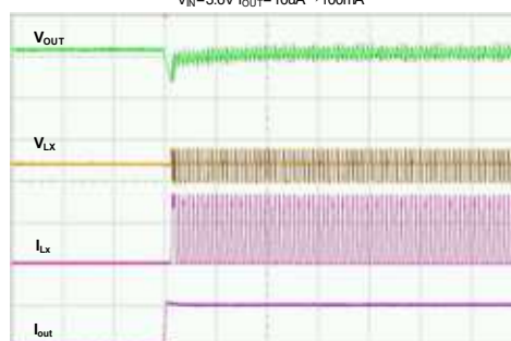
XC9265A181
