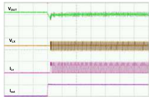
XC9265B181
