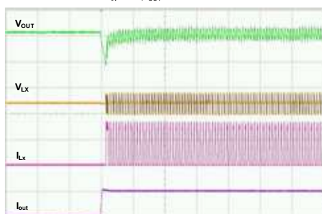
XC9265A181
