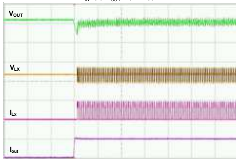
XC9265B181
