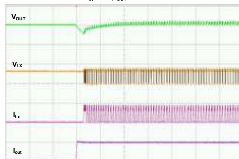
XC9265B301
