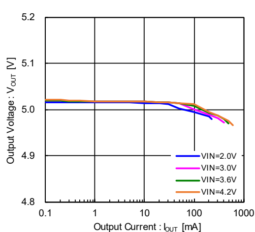
XCL103D503CR-G/XCL103E503CR-G
