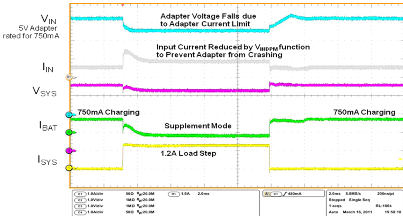
Figure 8. bq24270 V_{IN\_DPM}
