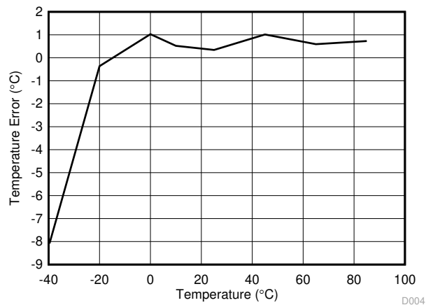
Figure 6-6. T_{(Err)}
