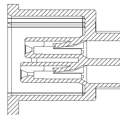
SECT A-A
