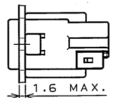
PANEL MOUNTED CONDITION(REF.) パネルマウント状態図(参考)
