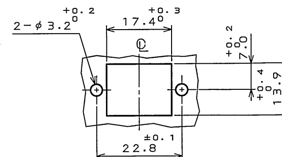
PANEL PATTERNS(REF.) パネル取付寸法(参考)
