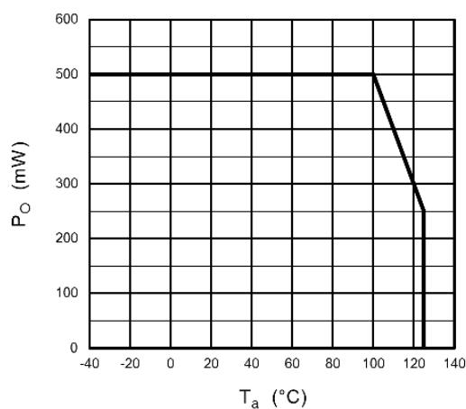
Fig. 13.2.3 P_O - T_a
