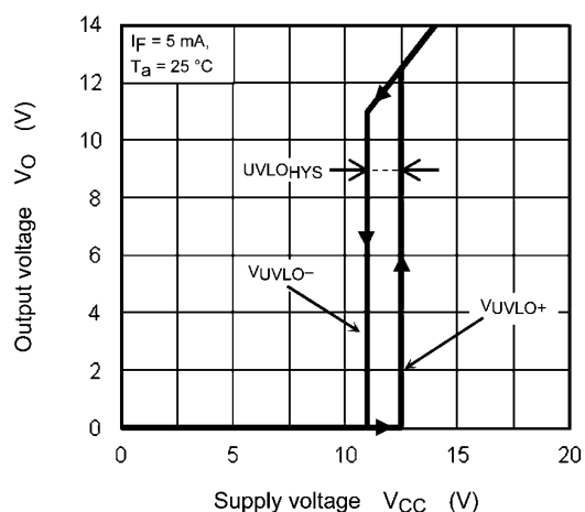
Fig. 13.2.11 V_O(V_{VLO}) - V_{CC}
