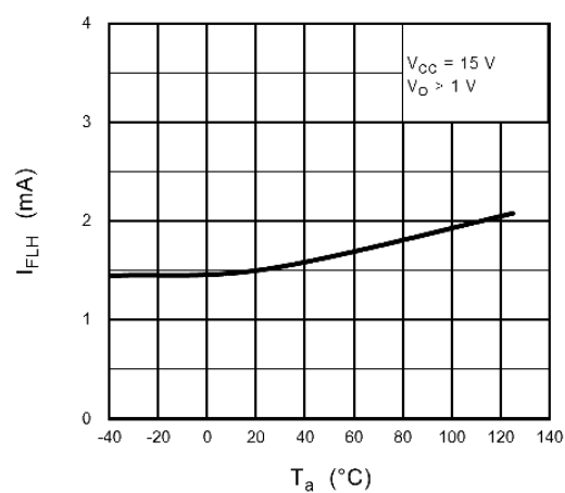
Fig. 13.2.4 I_{FLH} - T_a
