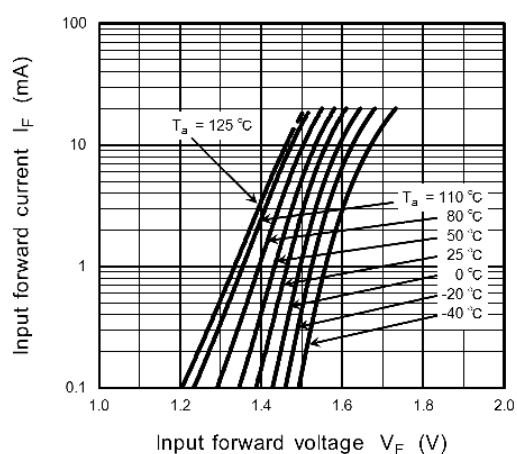
Fig. 13.2.1 I_F - V_F
