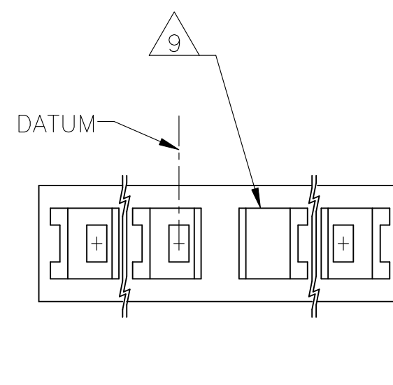
DETAIL Y
