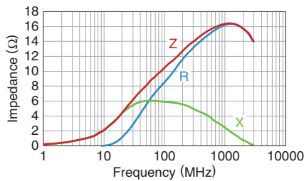
MPZ1005S100CTD25
