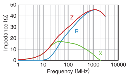
MPZ1005S300CTD25
