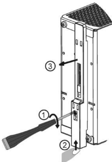
Fig. 3-2 Detach slide
