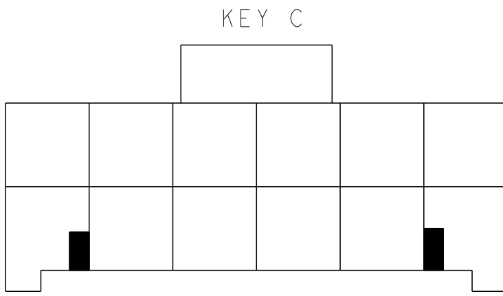
KEYING FOR 2*6 POS.
