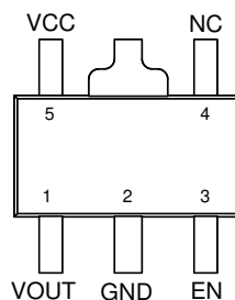
SOT-89-5
