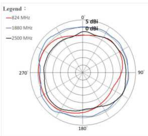
Elevation 1
