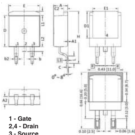
TO-263 Outline
