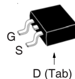
TO-263 (IXTA)
