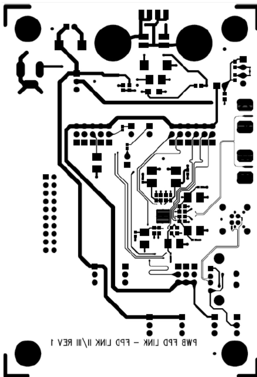
Figure 29. Bottom Layer
