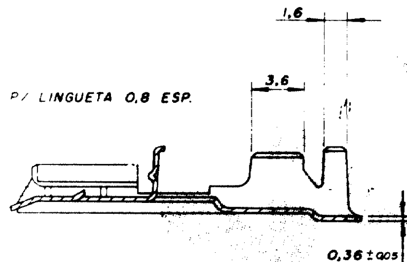
SEÇÃO "AA"
