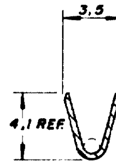
SEÇÃO "BB"
