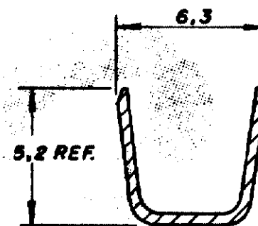
SEÇÃO "CC"
