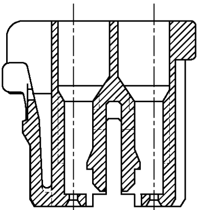
SECT A-A
