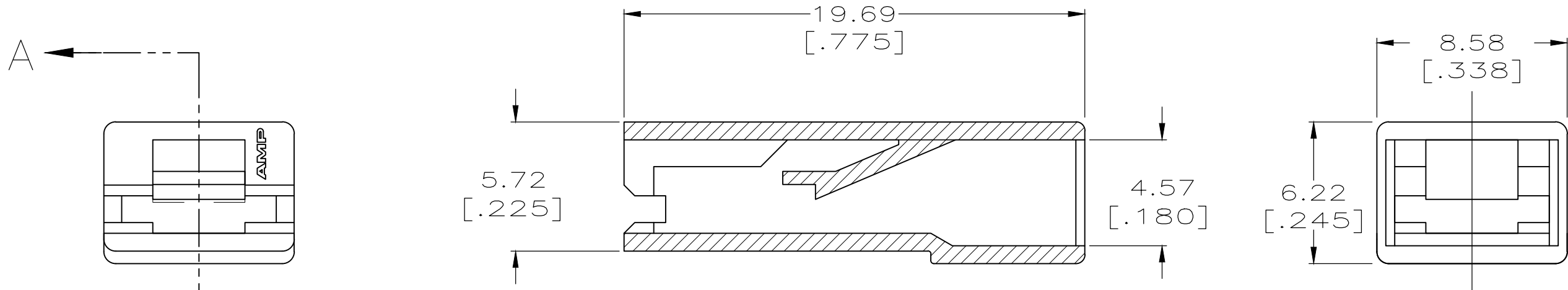
SECTION A-A
