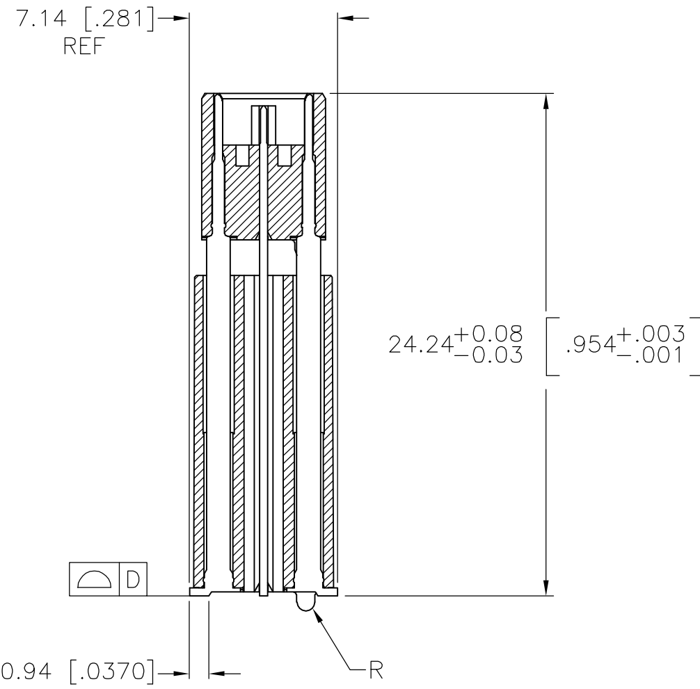
SECTION A-A
